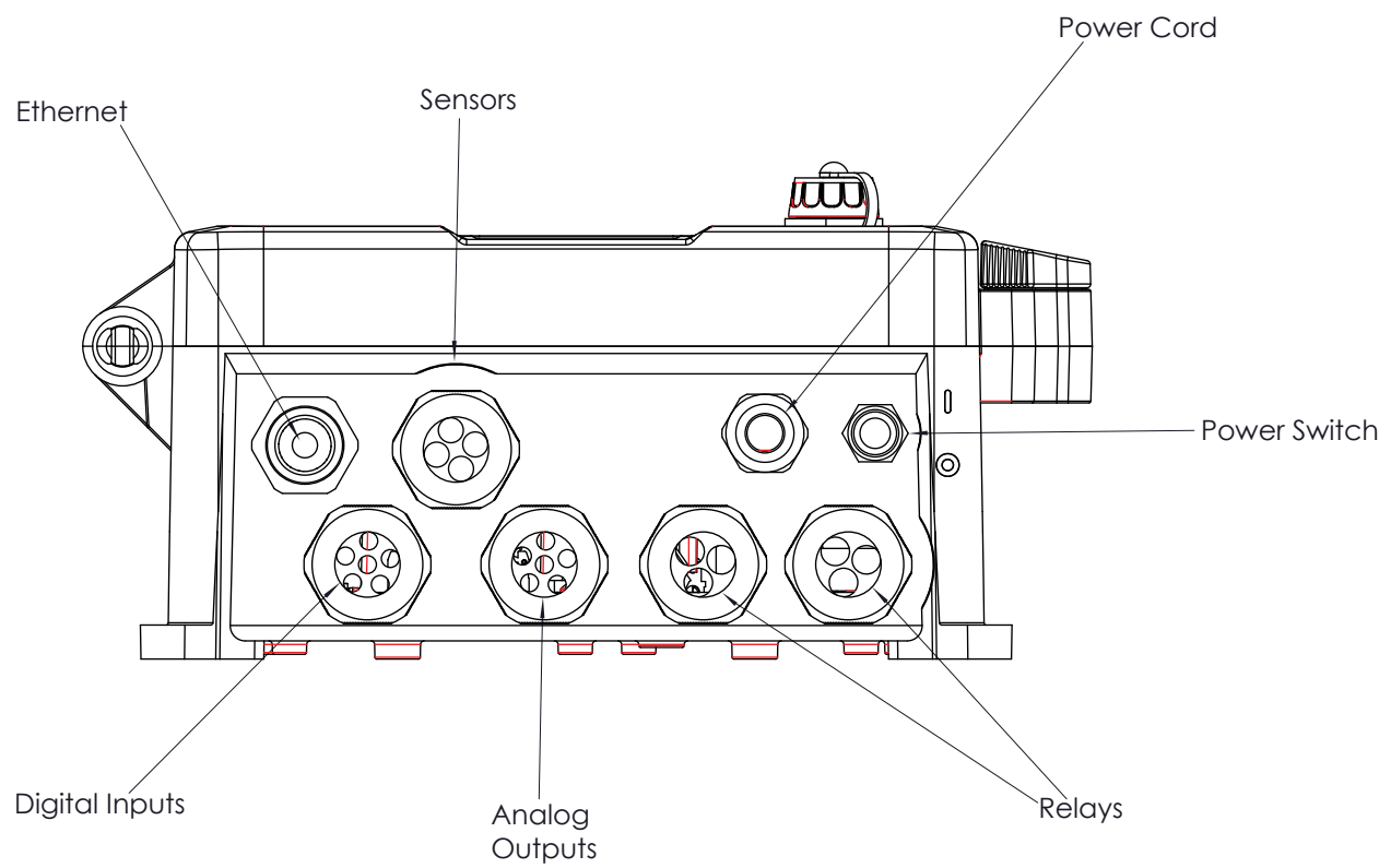
Figure 5 Conduit Wiring
